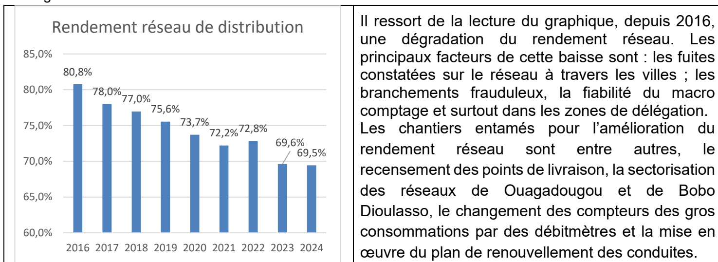
Figure 14: Evolution du rendement du réseau en milieu urbain
