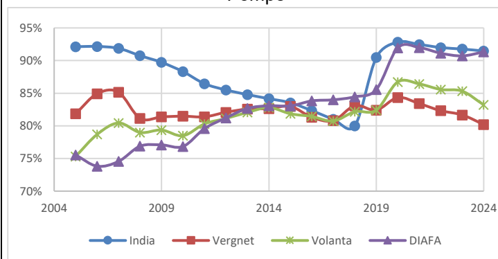
Figure 8: Taux de fonctionnalité des PEM selon le type de Pompe
