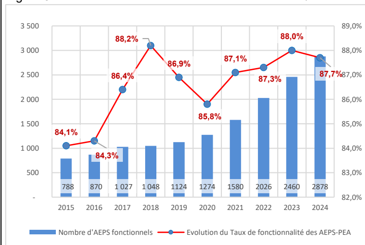
Figure 9: Evolution du Taux de fonctionnalité des AEPS/PEA
