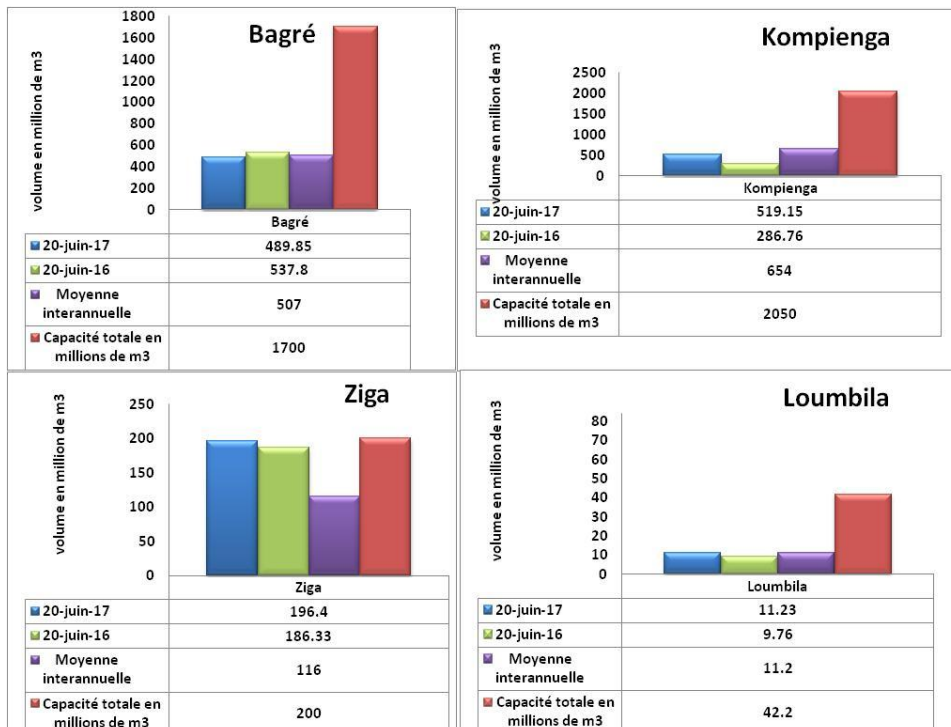
Figure 4: Situation de remplissage au 20 juin 2017, comparaison avec la situation de 2016, la moyenne inter-annuelle et la capacité nominale des barrages.
