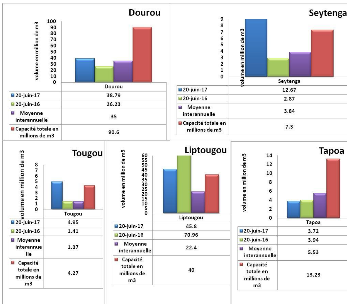
Figure 8: Situation de remplissage au 20 juin 2017, comparaison avec la situation de 2016, la moyenne inter-annuelle et la capacité nominale des barrages.
