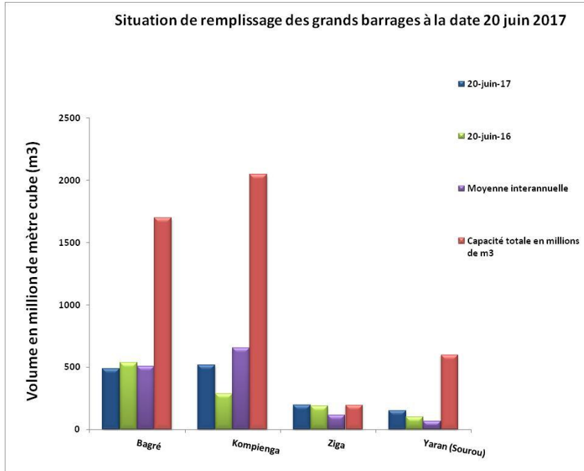
Figure 1: Situation de remplissage au 20 juin 2017, comparaison avec la situation de 2016, la moyenne inter-annuelle et la capacité nominale des barrages.
