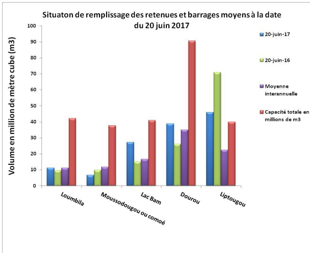
Figure 2: Situation de remplissage au 20 juin 2017, comparaison avec la situation de 2016, la moyenne inter-annuelle et la capacité nominale des barrages.
