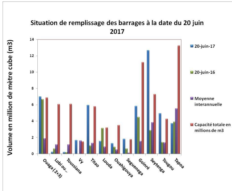
Figure 3: Situation de remplissage au 20 juin 2017, comparaison avec la situation de 2016, la moyenne inter-annuelle et la capacité nominale des barrages.
