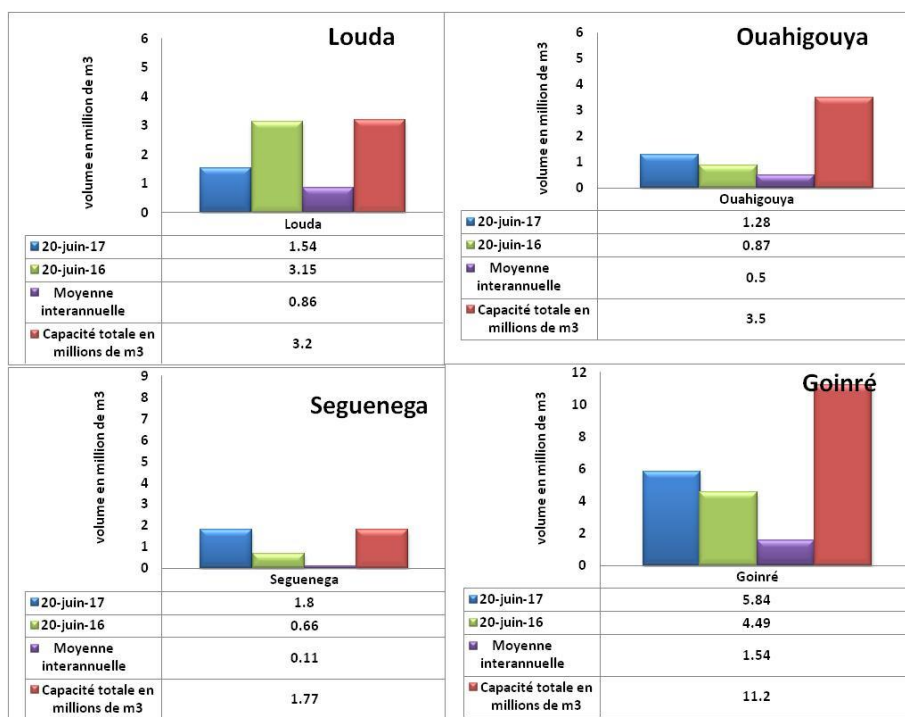
Figure 7: Situation de remplissage au 20 juin 2017, comparaison avec la situation de 2016, la moyenne inter-annuelle et la capacité nominale des barrages.
