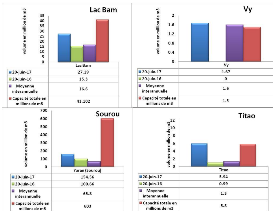
Figure 6: Situation de remplissage au 20 juin 2017, comparaison avec la situation de 2016, la moyenne inter-annuelle et la capacité nominale des barrages.
