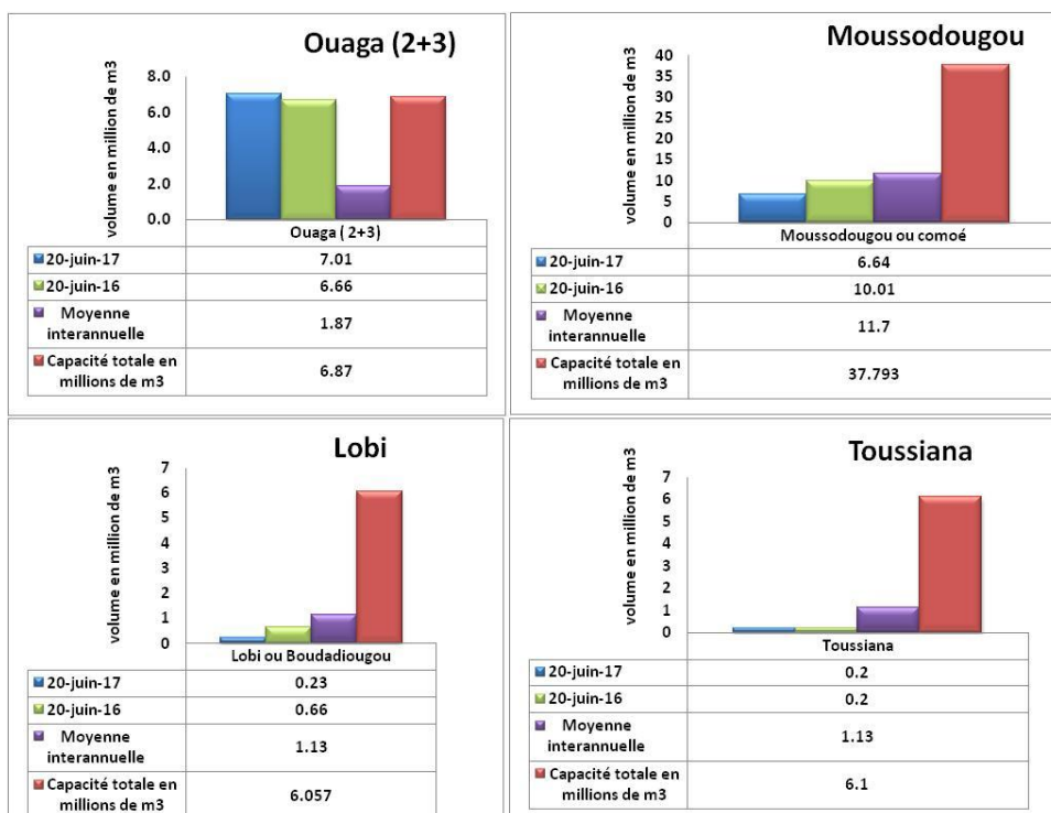
Figure 5: Situation de remplissage au 20 juin 2017, comparaison avec la situation de 2016, la moyenne inter-annuelle et la capacité nominale des barrages.
